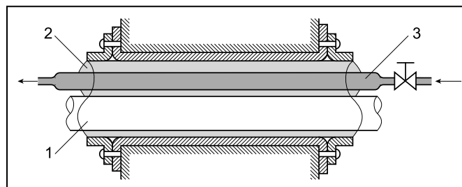
Rys. 13.2. Przykład rozwiązania konstrukcyjnego układu do chłodzenia kabla energetycznego przepływającym czynnikiem chłodzącym 1 – rdzeń kabla, 2 – olej kablowy, 3 – przewód chłodzący
